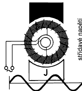
Schéma alternátoru: J jižní pól elektromagnetu
