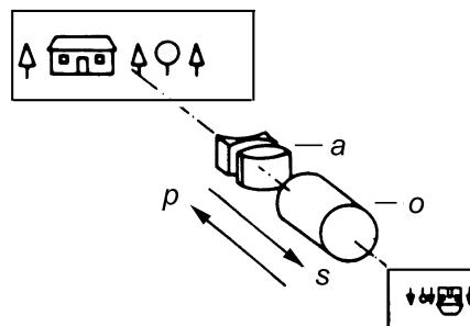
Schéma anamorfotického zobrazování v kinematografii: a anamorfotická předsádka, o objektiv, s snímání, p promítání
