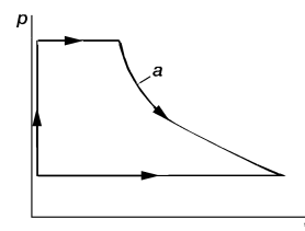
Průběh adiabaty pro dokonalý děj, a adiabatická expanze, p tlak, v objem
