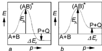
Změny energie E v průběhu přeměny dvojice molekul A a B na dvojici molekul P a Q. Při přeměně se energie a uvolňuje ( \Delta E_r < 0 ); b spotřebává ( \Delta E_r > 0 ); p průběh reakce, (AB)^* aktivovaný komplex, E_a aktivaci energie, \Delta E_r reakční energie
