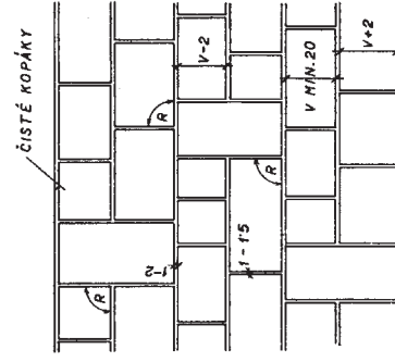
LÍČ SVISLE PROVAZOVANÉHO ČISTÉHO ZDIVA RÁDKOVÉHO.
