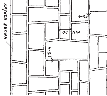
LÍČ SVISLE PROVAZOVANÉHO HRUBĚHO ZDIVA RÁDKOVÉHO.
