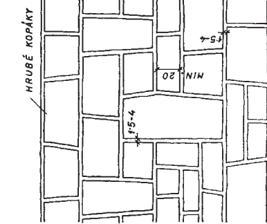
LÍČ SVISLE PROVAZOVANÉHO HRUBĚHO ZDIVA RÁDKOVÉHO.
