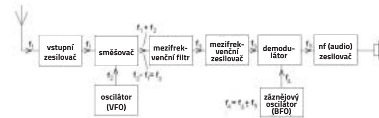
Blokové schéma superhetu
