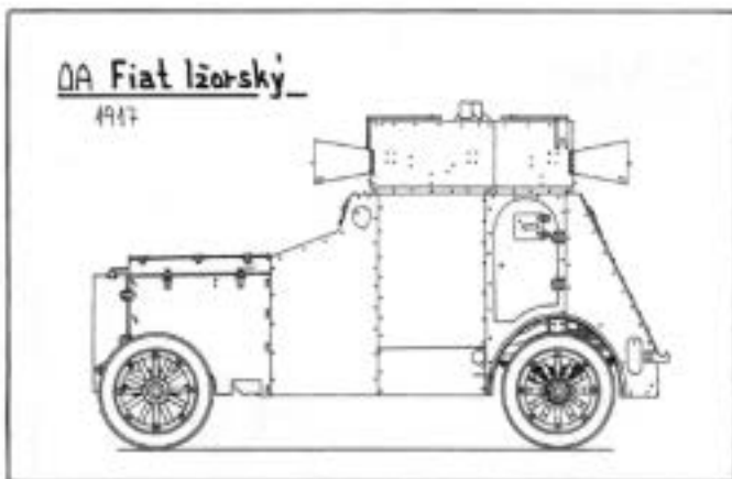
Ruský obrněný automobil Fiat, opancěrovaný v Ižorském závodě (nákres J. Suchý)
