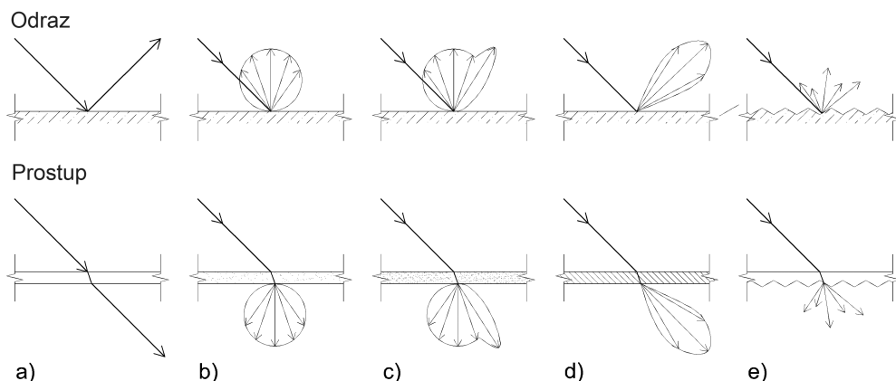
Obr. 2.3.1 Světelný odraz a prostup směrového paprsku
