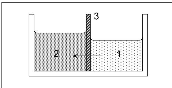
Obr. 1-2 Osmóza
