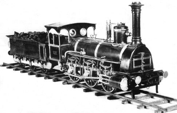
Obr. 4 Model lokomotivy Ernst Turnovsko-kralupsko-pražské dráhy od jejího strojevodoucího Macana
