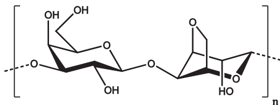
agaróza
