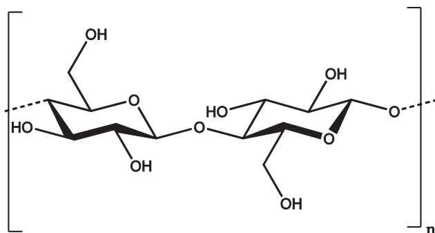
celulóza
