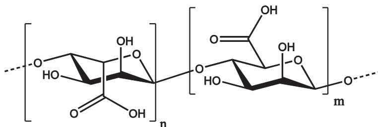
kyselina alginová
