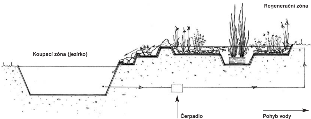
obr. 11 Jednodílnové koupací jezírko
