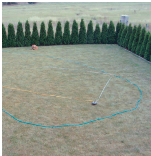
obr. 12 Vyměření tvaru koupacího jezírka
