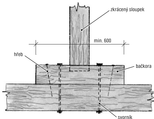
Obr. 13 Oprava sloupku pomocí podložky s dlabem
