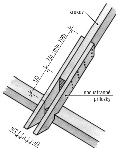
Obr. 10 Oprava uhnílého spodního konce krovce pomocí příložek
