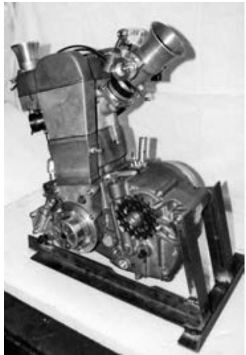
Detail nového čtyřdobého jednoválce Ahra 800 TOHC
