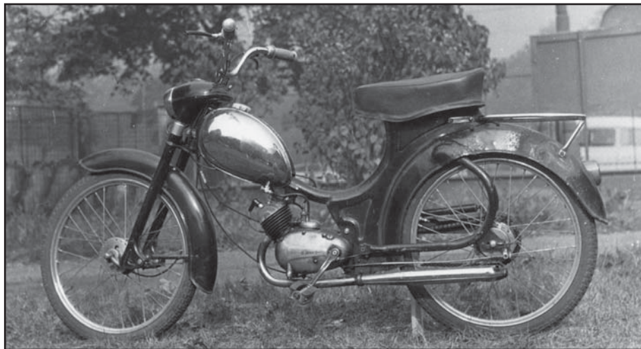
Prototyp č. 02 byl kompletně celý v černém lakování a objevil se u něj problém s únavovým praskáním zadního blatníku, v místech za kapsami pro oblouk vidlice. Blatník i po zavaření praskal znovu a znovu. Na snímku je opravované a překlepávané místo zřetelné.
