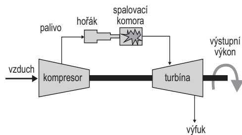
Obr. 2.1 Princip práce spalovací turbíny [16]
