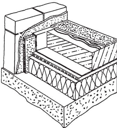
Obr. 3.12 Řez modulovou klima-podlahou
